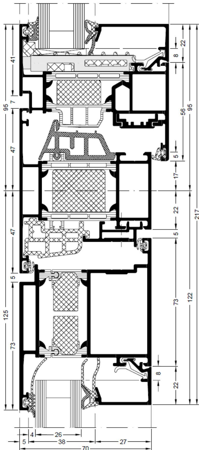
Detail oben Flügel/ Kämpfer/ Kippflügel einwärts öffnend
