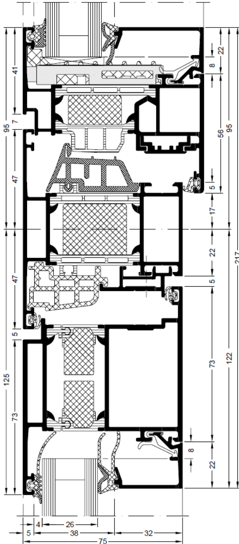
Detail oben Flügel/ Kämpfer/ Kippflügel einwärts öffnend
