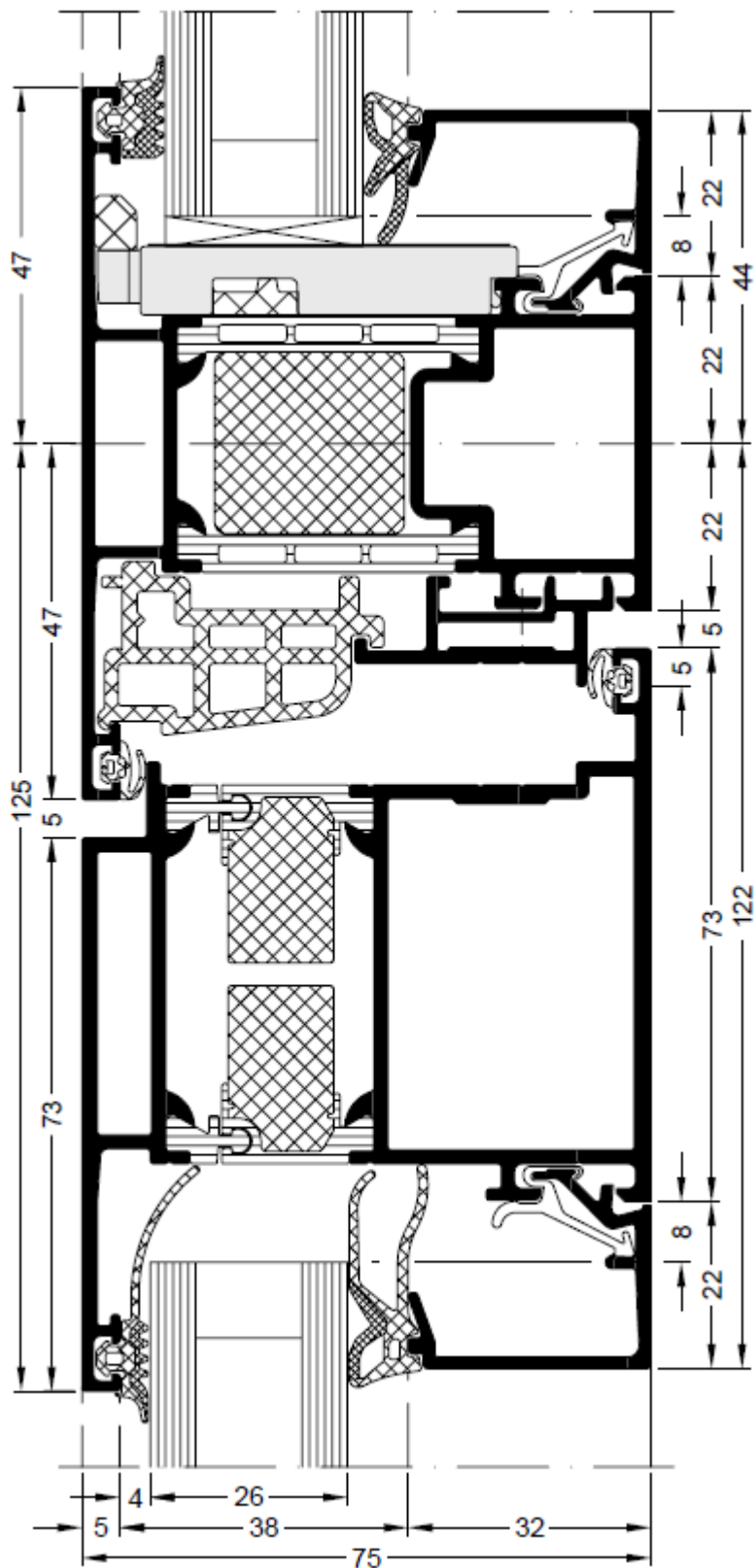
Detail oben Flügel/ Kämpfer/ Oblicht einwärts öffnend
