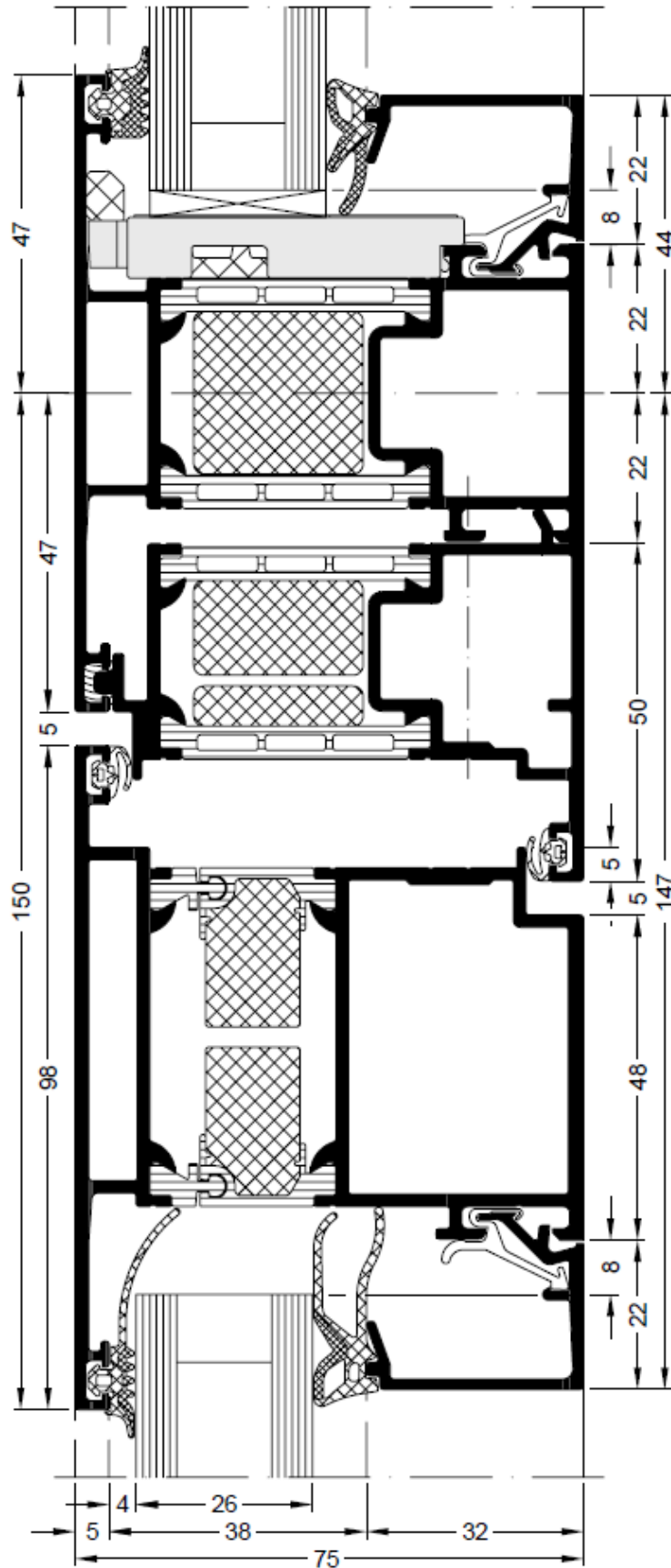
Detail oben Flügel/ Kämpfer/ Oblicht auswärts öffnend
