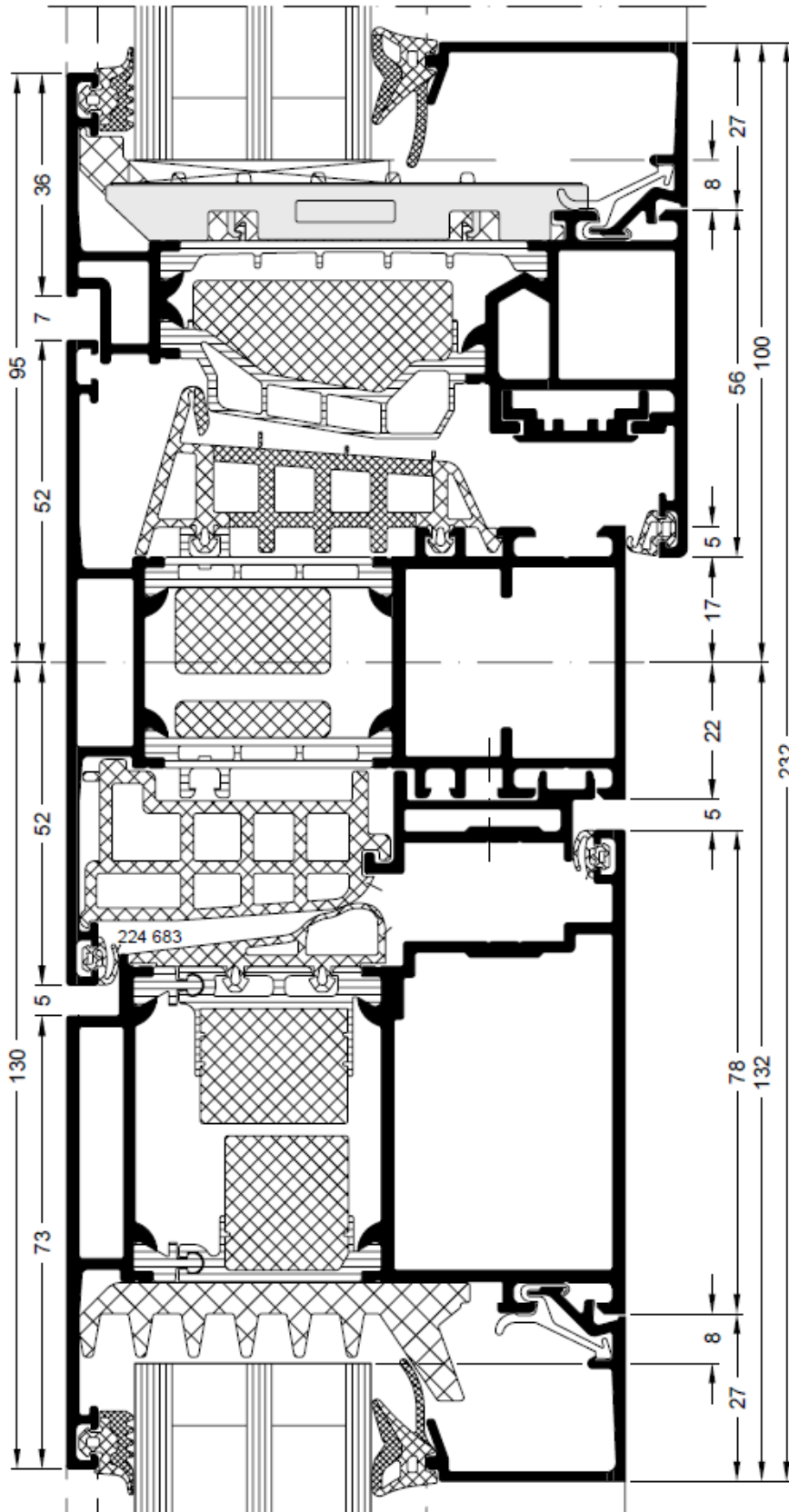
Detail oben Flügel/ Kämpfer/ Kippflügel einwärts öffnend
