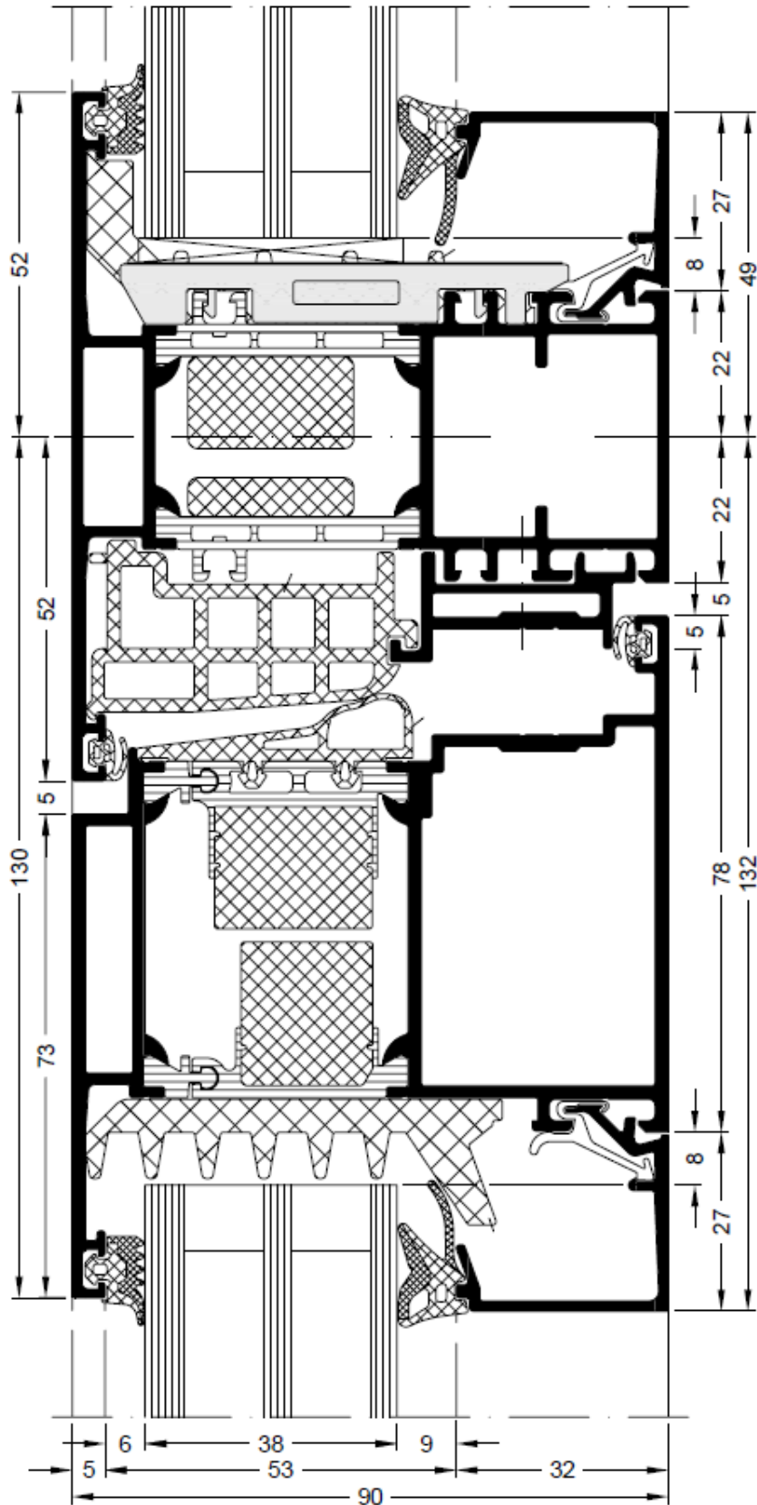
Detail oben Flügel/ Kämpfer/ Oblicht einwärts öffnend
