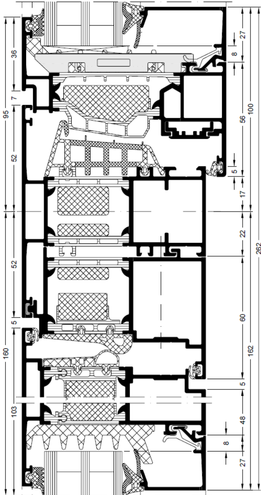
Detail oben Flügel/ Kämpfer/ Kippflügel auswärts öffnend
